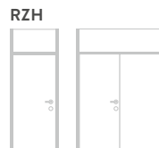
Raumhohe Zarge ohne Querteil mit Kämpfer und Oberlichte (einflügelig, zweiflügelig)
